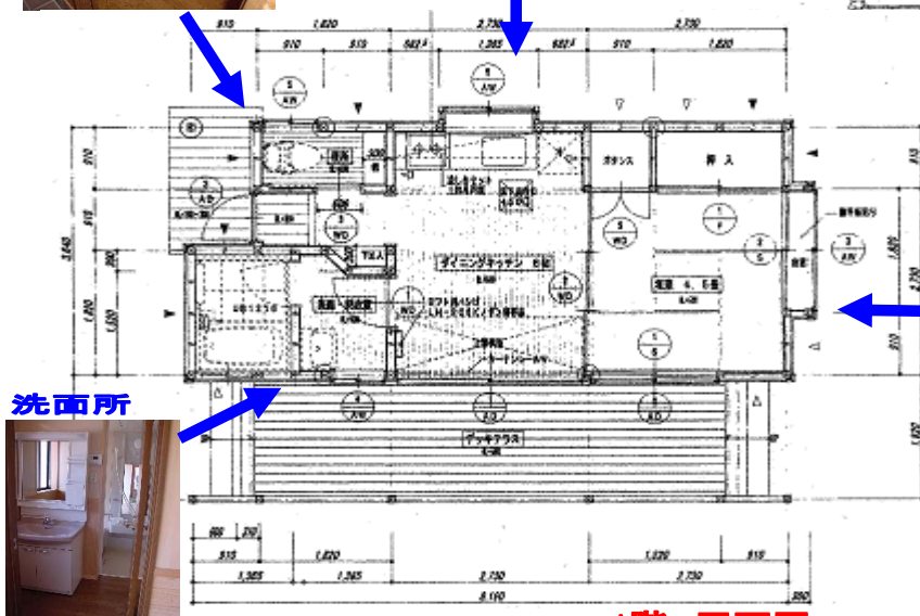
1階 平面図
